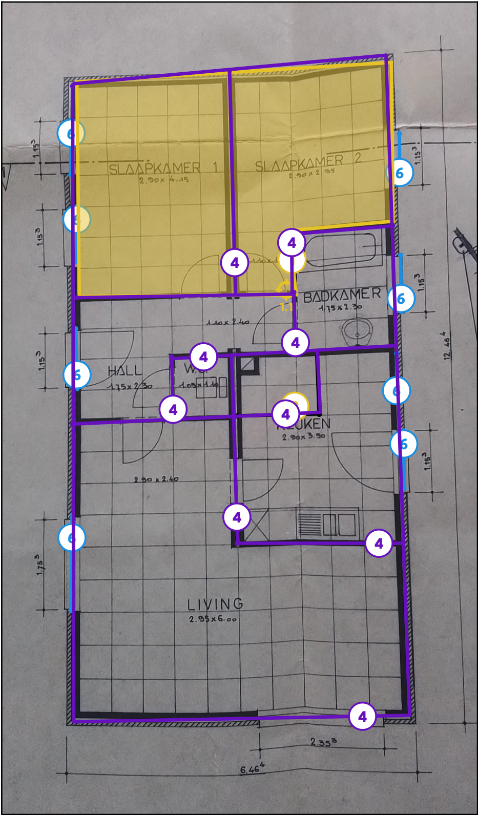
Legende van plan 1.2: Gelijkvloers, mastiek, vloerzeil, pleisterwerk
